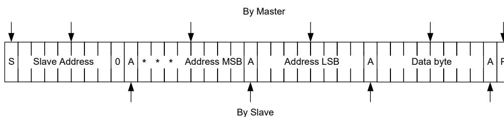
Fig. 4: single byte write
