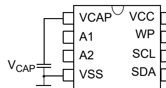
Fig. 10: PowerStore Cofiguration
